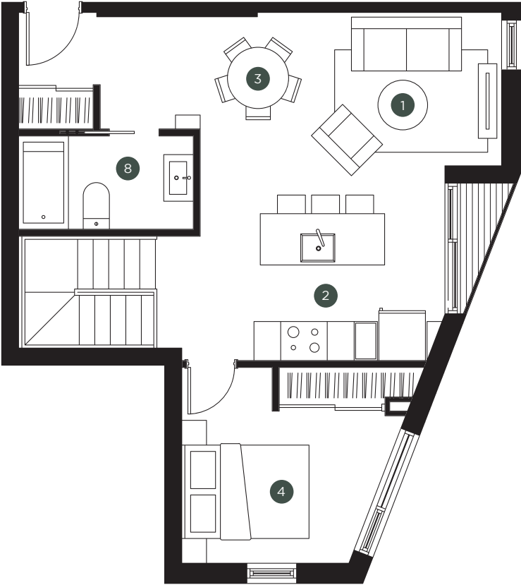
ÉTAGE 1 / LEVEL 1
